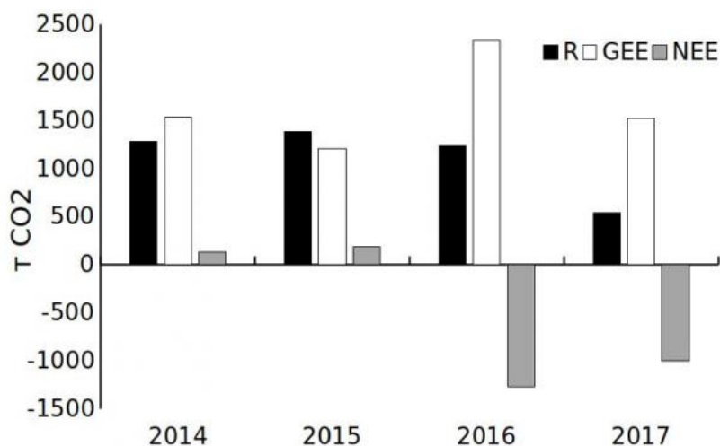
Рисунок 1 – Интегральные потоки \text{CO}_2 со всей площади ГМК за летние периоды
