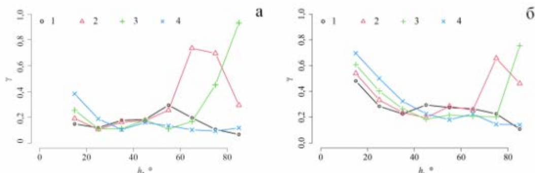
Рисунок 2 – Зависимости коэффициента пропускания \gamma излучения пологом от угловой высоты приемника излучения h при разной величине смещения m очага горения относительно крон для случая прохождения излучения через массив из трех крон-эллипсоидов Populus tremula с диаметром 3 м и отношением длин полуосей 4:3:3 (а) и 8:3:3 (б) при ЛИ = 2,5; 1 – m = 0 м, 2 – m = 1,0 м, 3 – m = 2,0 м, 4 – m = 3,0 м
