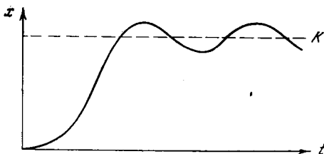
Рис. 7. Динамика популяции при учете временного запаздывания
