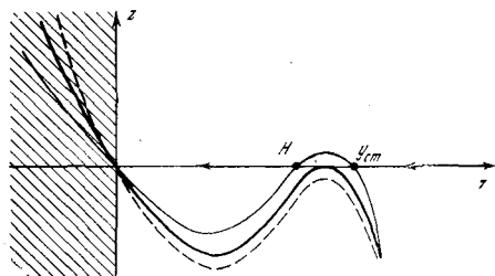
Рис. 2. Точка А. Жесткий срыв колебаний
