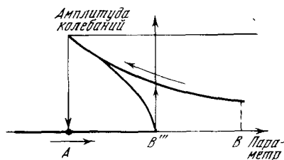
Рис. 12. Срыв колебаний при растущей амплитуде
