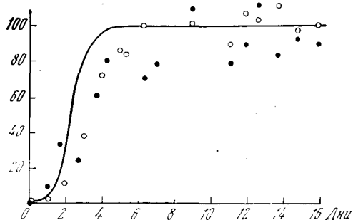
Рис. 1. Рост изолированных популяций P. aurelia и P. caudatum (Гаузе, 1934)
