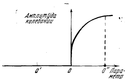
Рис. 9. Граница мягкого и жесткого режимов
