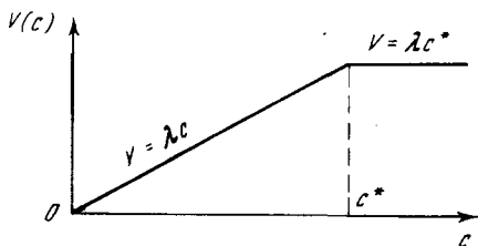
Рис. 3. Конкретный вид функции выедания V(c)
